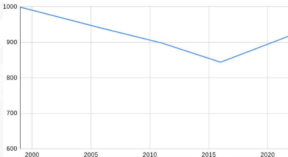
Evolution de la population de Pardies depuis 2000
